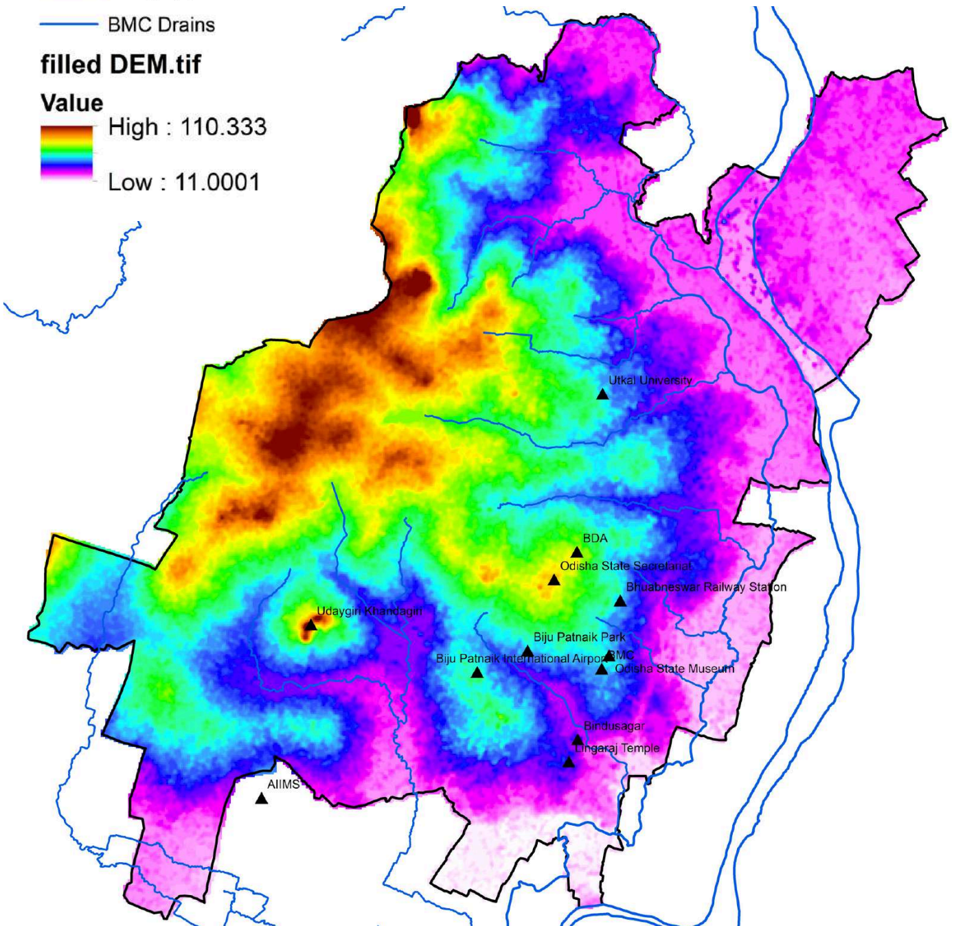
Elevation
